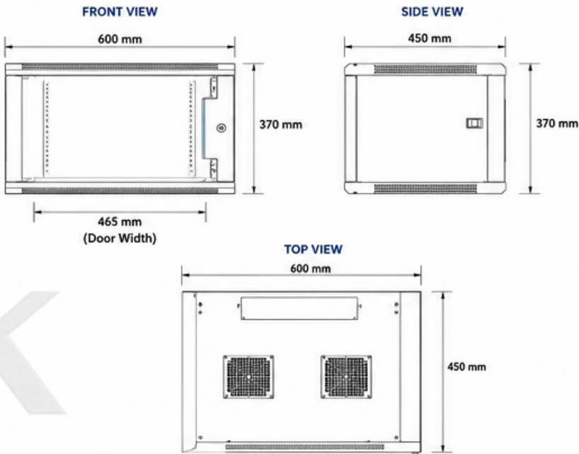
DIMENSIONS
